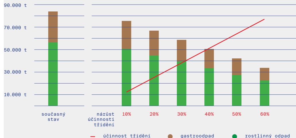
Obrázek 9: Potenciál snížení hmotnosti organických odpadů v SKO. Zdroj: Prognóza PSAS (2021)
